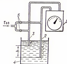
Рис. 2. Схема дифференциального гидростатического плотномера с продувкой газа: 1 — дифференциальный манометр; 2 — длинная трубка; 3 — короткая трубка; 4 — сосуд с исследуемой жидкостью; 5 — вентили.
